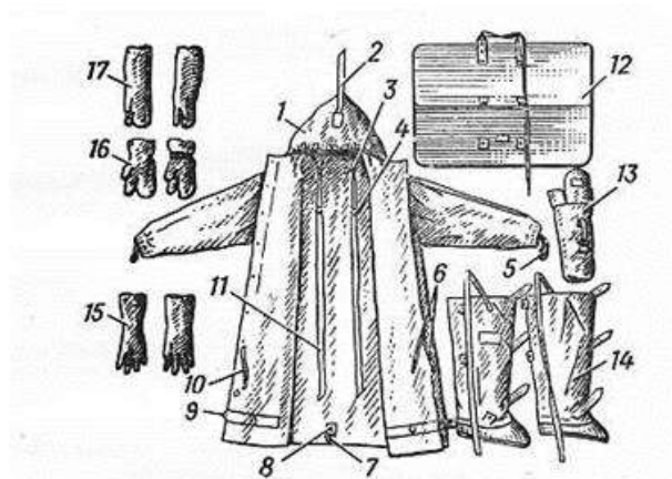
Рис. 6.1. Общевойсковой защитный комплект: 1 — защитный плащ ОП-1М; 2 — застежка; 3 — петли спинки; 4 и 7 — рамки стальные; 5 — петля для большого пальца руки; 6 и 10 — за- перки; 8 — центральный шлевек; 9 — хвостик; 11 — держатель пла- ща; 12 — чехол для защитного плаща ОП-1М; 13 — чехол для защит- ных чулок и перчаток; 14 — защитные чулки; 15 — защитные перчатки БЛ-1М; 16 — утеплительные вкладыши к защитным перчаткам БЗ-1М; 17 — защитные перчатки БЗ-1М
